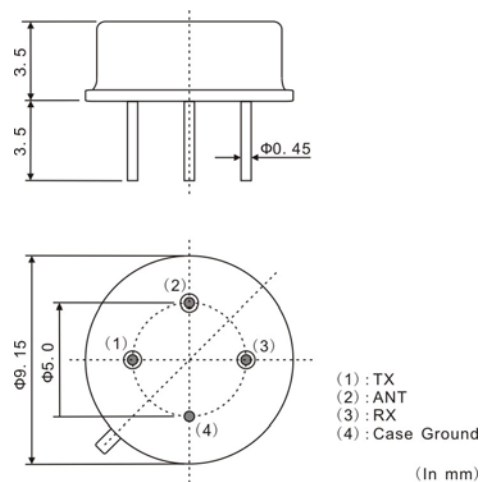
TO39B
