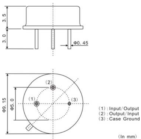
TO39A
