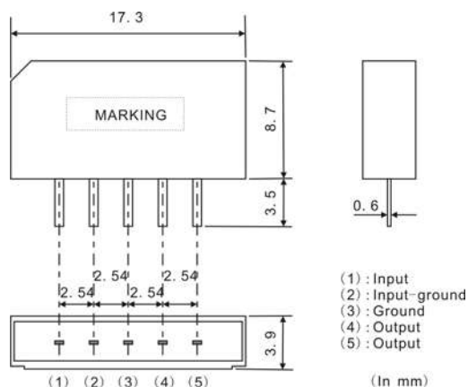
SIP5K
