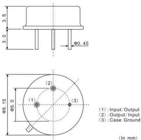
TO39A
