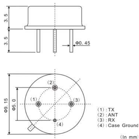
TO39B
