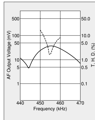
CDBC455CX32/TA31143
