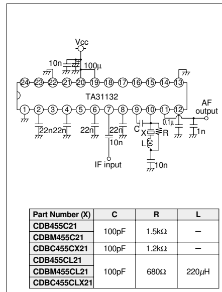
TA31132
